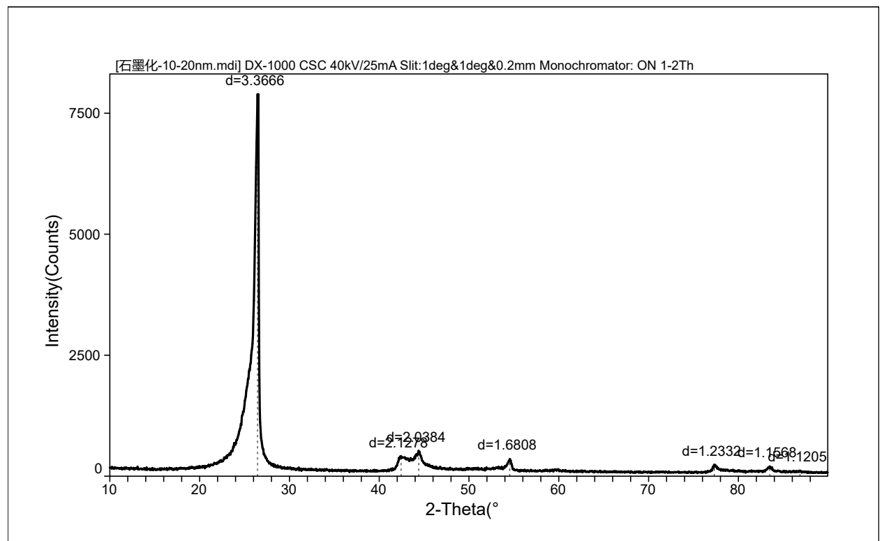
XRD
